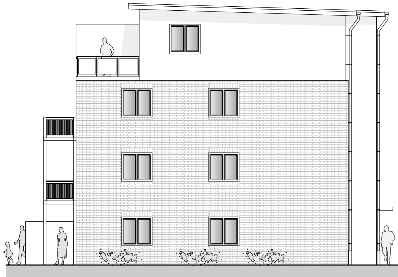
ANSICHT OSTEN
