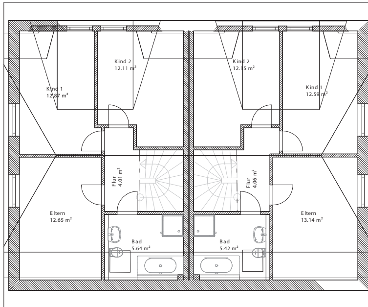
Dachgeschoss
